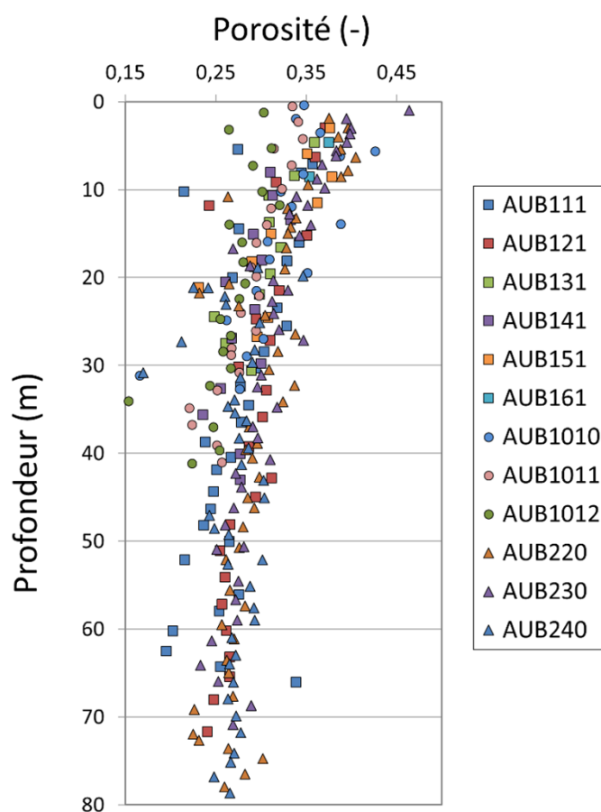
Figure 4-16 Évolution de la porosité totale des Argiles téglines en fonction de la profondeur
