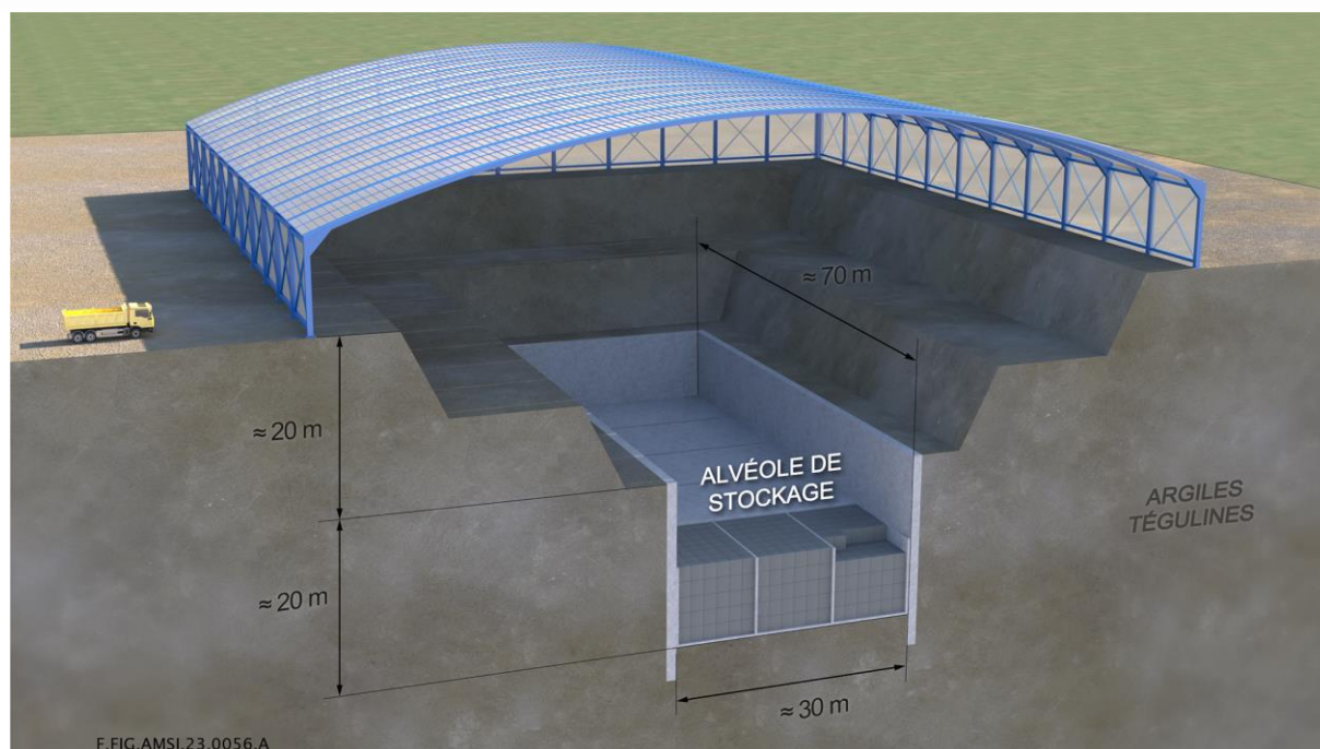
Figure 7-4 Illustration d'un ouvrage de stockage à ciel ouvert mixte : terrassement et soutènement linéaire vertical (exemple avec 10 m de hauteur de stockage)
