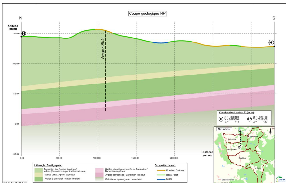
Figure 4-8 Coupe géologique nord-sud au nord du secteur d'étude
