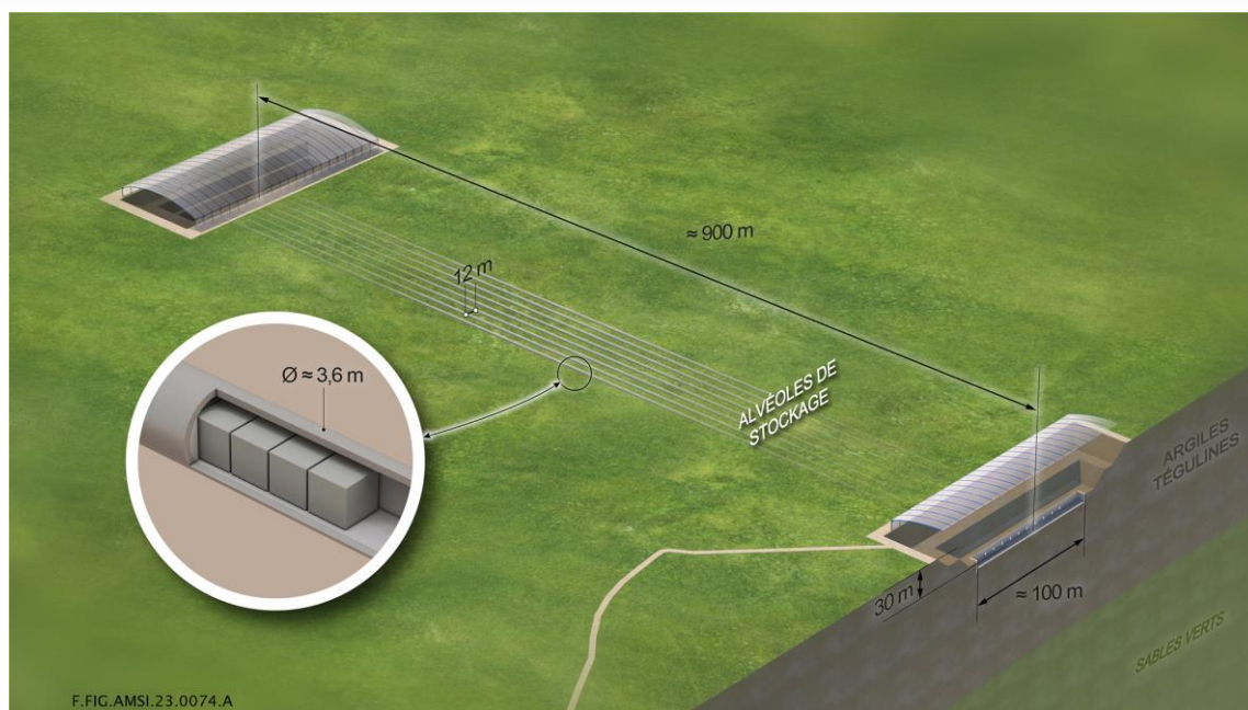
Figure 7-7 Illustration d'un module de stockage composé d'une dizaine d'alvéoles de l'ordre de 3 m de diamètre utile réalisés par microtunnelier avec accès par tranchées sous abri
