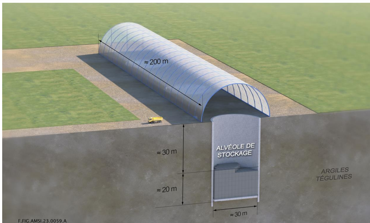
Figure 7-3 Illustration d'un ouvrage de stockage réalisé en soutènement linéaire vertical type puits depuis la surface (exemple avec 20 m de hauteur de stockage)
