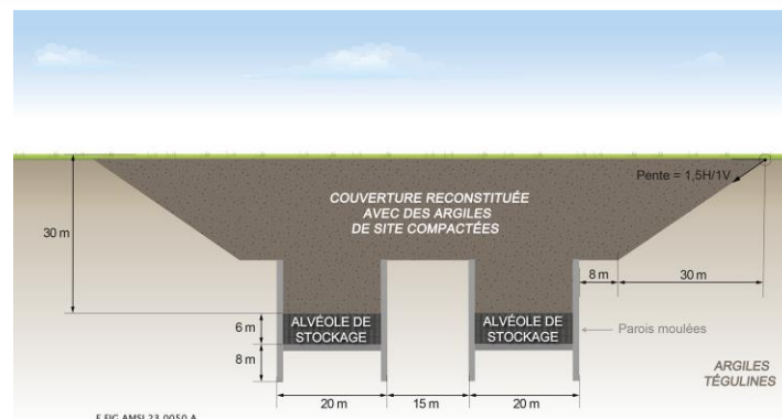
Figure 7-9 Illustration de l'architecture de stockage à ciel ouvert étudiée pour les évaluations de sûreté après-fermeture
