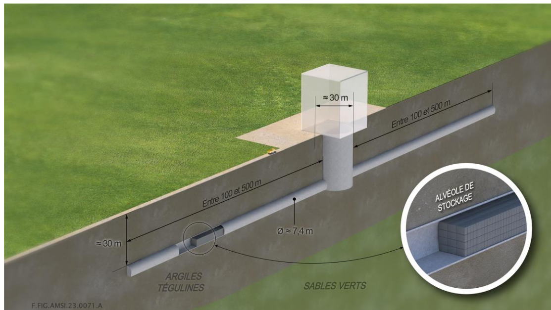
Figure 7-5 Illustration d'un module de stockage de deux alvéoles, réalisé par creusement conventionnel (diamètre excavé de l'ordre de 10 m) avec un accès par puits sous abri
