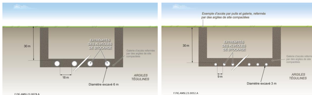
Figure 7-8 Illustration des architectures de stockage en souterrain étudiées pour les évaluations de sûreté après-fermeture
