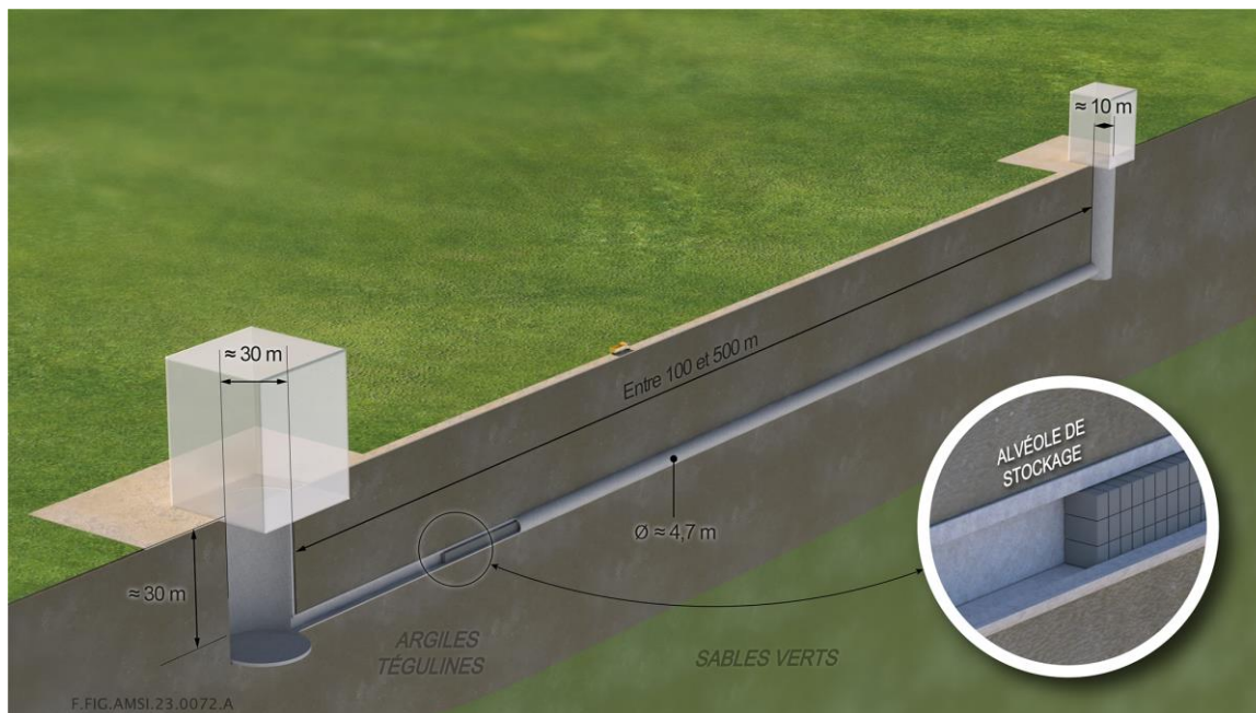
Figure 7-6 Illustration d'un module de stockage composé d'un alvéole de stockage de l'ordre de 5 m de diamètre utile réalisé par tunnelier avec accès par puits sous abri
