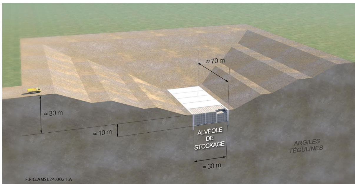
Figure 7-1 Illustration d'un ouvrage de stockage réalisé en terrassement pleine fouille jusqu'au toit du stockage (exemple avec 10 m de hauteur de stockage)
