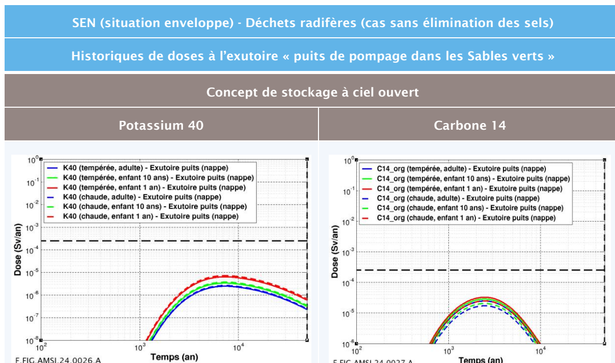
Figure 8-6 SEN - situation enveloppe, déchets radifères (cas sans élimination des sels), potassium 40 et carbone 14 : historiques de doses à l'exutoire « puits de pompage dans les Sables verts » pour le concept de stockage à ciel ouvert, pour les biosphères tempérée et chaude et les classes d'âge adulte et enfant (10 ans, 1 an)
