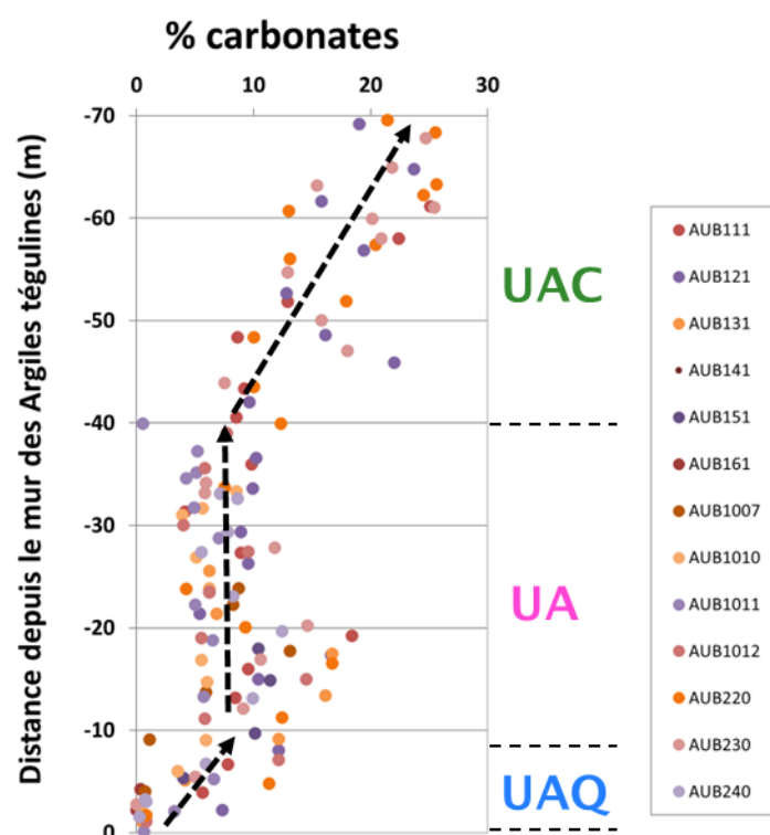
Figure 4-15 Évolution de la teneur en carbonates dans les Argiles téglines (distance à partir du mur de la couche)
