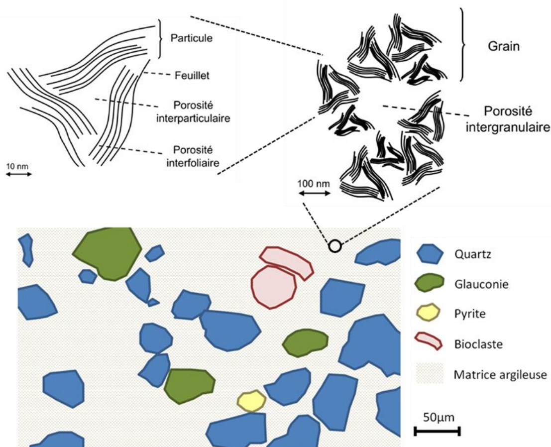
Figure 4-17 Représentation conceptuelle des arrangements minéraux dans les Argiles tégulines
