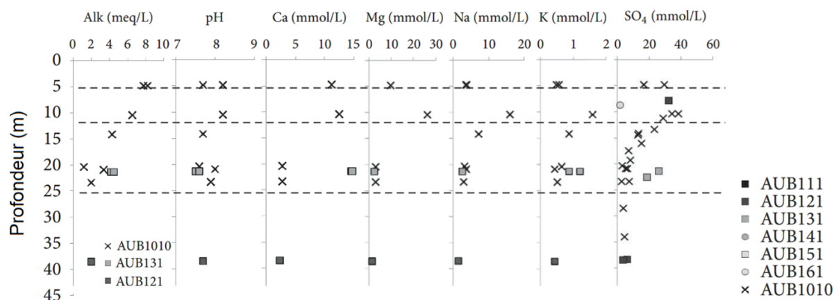
Figure 4-18 Évolution de la chimie des eaux des Argiles téglines en fonction de la profondeur pour différents forages (Alk : alcalinité)
