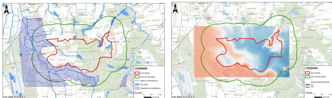
Figure 6-2 Zones artésiennes (à gauche), gradients hydrauliques (à droite)
