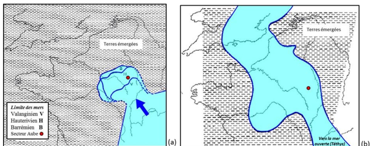
Figure 4-6 Évolution de l'extension des incursions marines, du Valanginien (a) à l'Albien (b) (schéma modifié d'après Collete et al., 1995)
