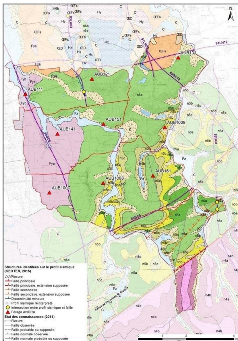
Figure 4-11 Schéma structural du secteur d'étude (réalisé en 2015)
