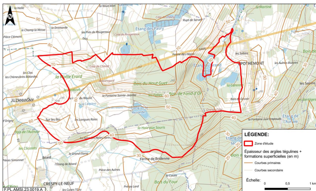
Figure 9-2 Carte représentant les profondeurs du mur de la couche des Argiles tégulines
