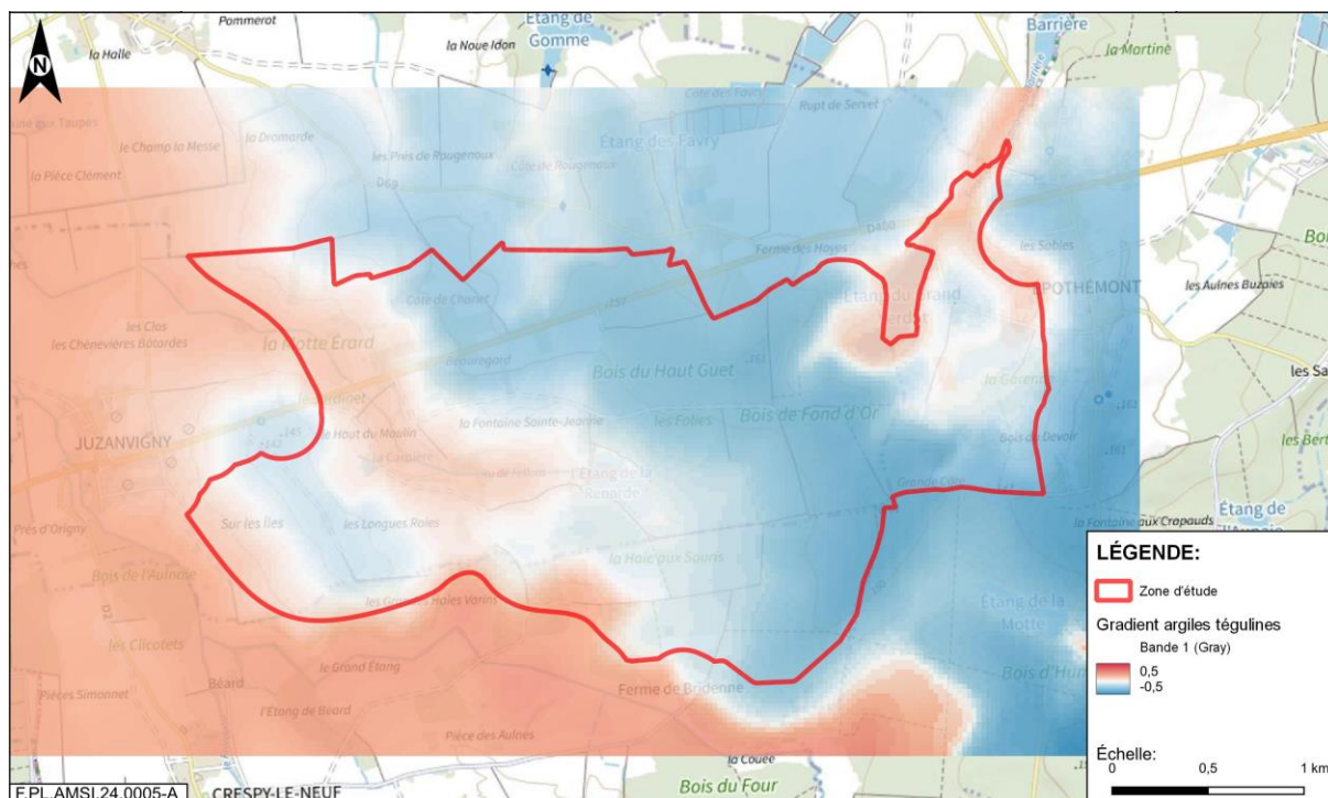
Figure 4-23 Carte de distribution spatiale du gradient de charge hydraulique vertical à travers les Argiles téglines sur la zone d'étude et alentour
