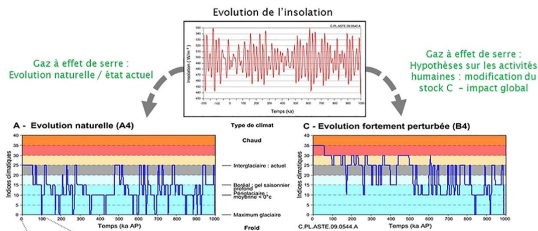
Figure 4-24 Scénarios d'évolution du climat sur le prochain million d'années
