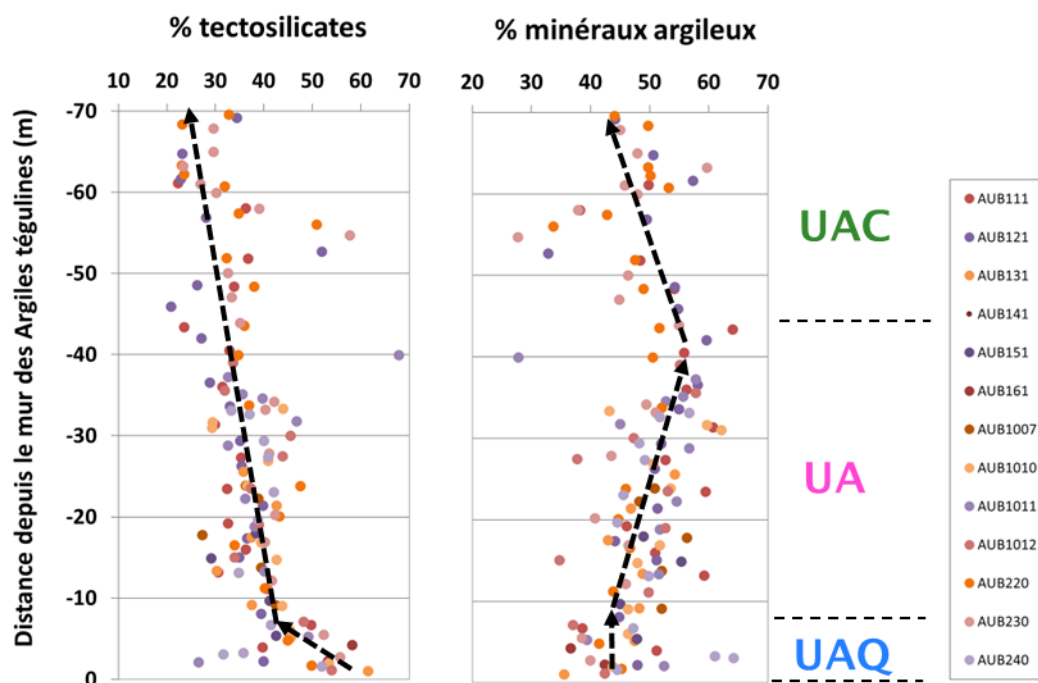
Figure 4-14 Évolution de la teneur en minéraux argileux et en tectosilicates dans les Argiles téglines (distance à partir du mur de la couche)
