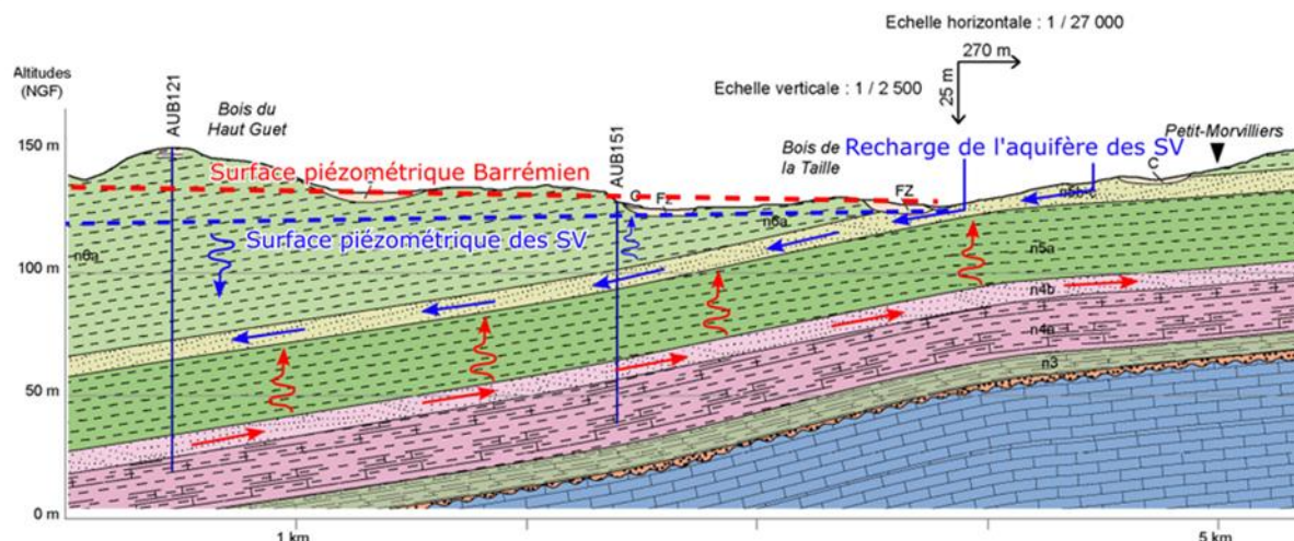
Figure 4-22 Schéma conceptuel selon une coupe nord-sud des écoulements de l'aquifère des Sables verts et du Barrémien sur le secteur d'étude
