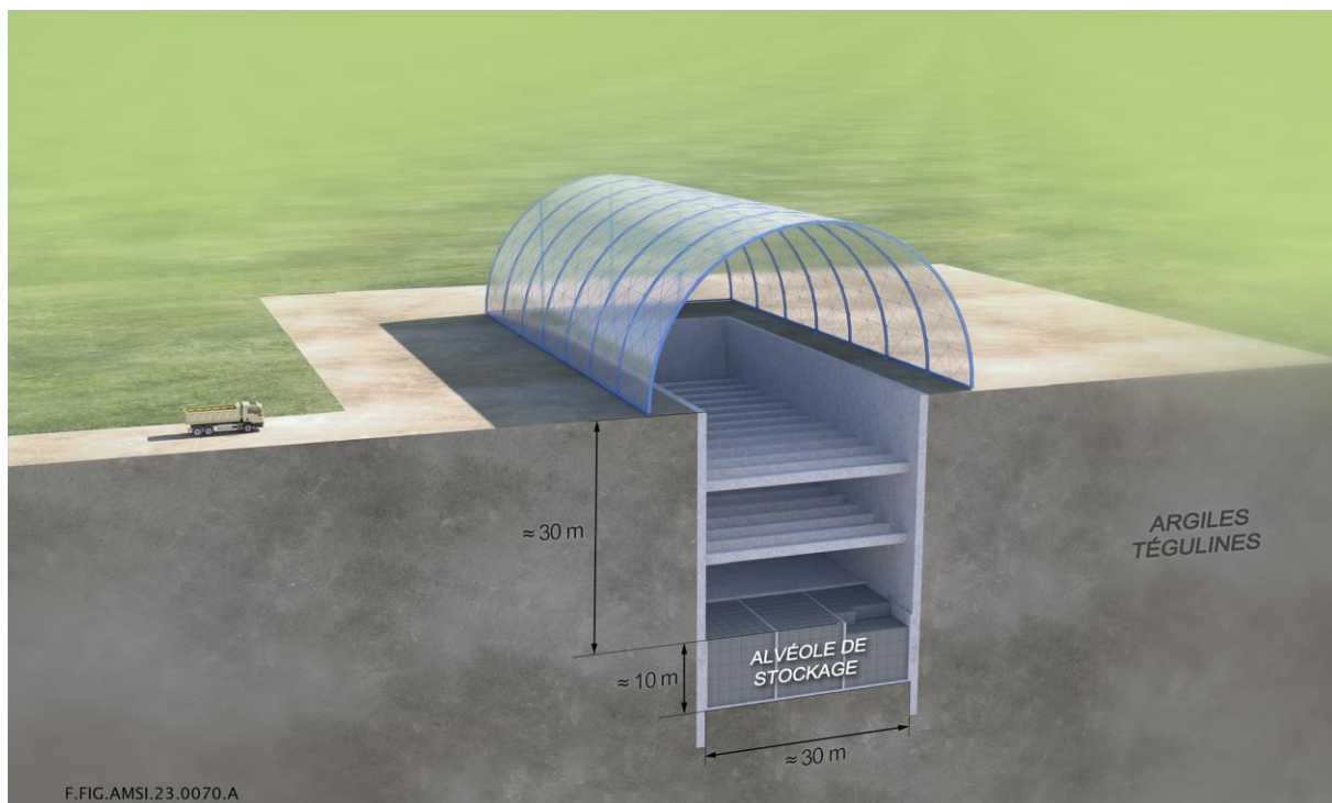
Figure 7-2 Illustration d'un ouvrage de stockage réalisé en soutènement linéaire vertical depuis la surface (exemple avec 10 m de hauteur de stockage)
